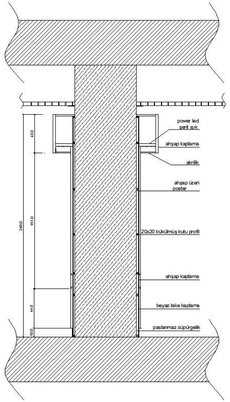
DÜŞEY 1-1 KESİTİ
