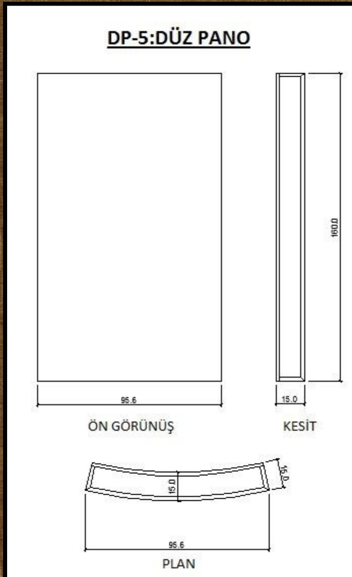
DP-5 : 15 x 96 x 160(h)
