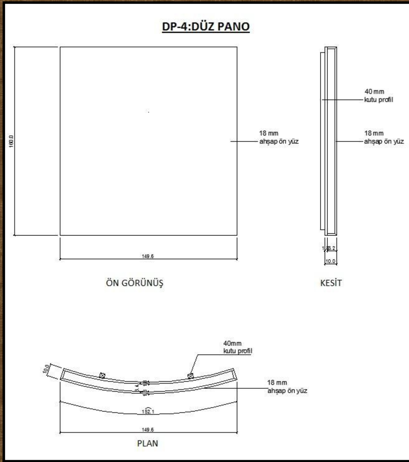
DP-4: 10 x 150 x 160(h)
